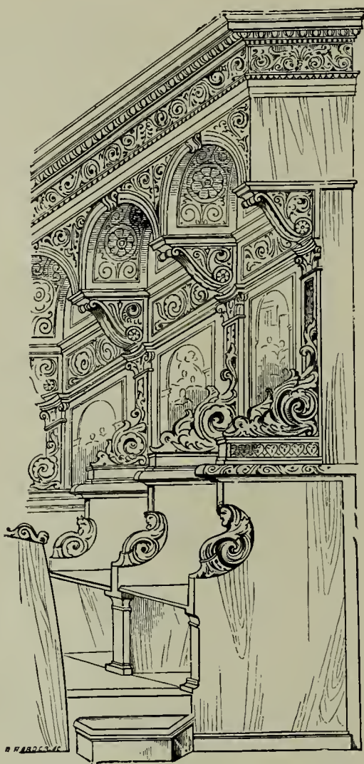
Abb. 303. Chorstühle aus S. Giovanni in Parma. (Nohl.)
